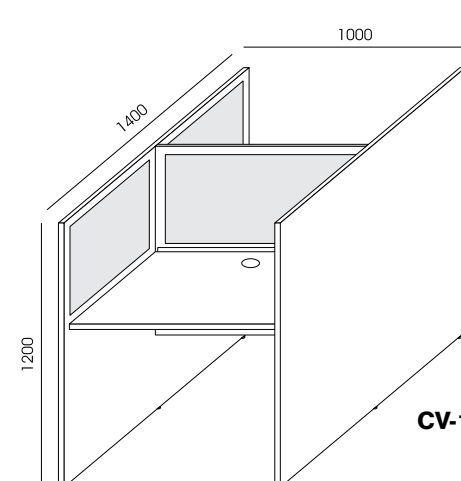
BASE MODULE
