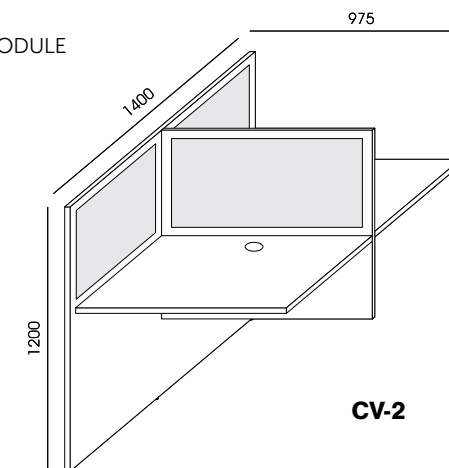
EXTENSION MODULE
